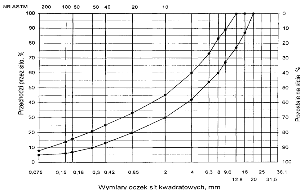
Rys. 4. Krzywe graniczne uziarnienia mieszanki mineralnej BA od 0 do 16 mm do warstwy wyrównawczej nawierzchni drogi o obciążeniu ruchem KR3
