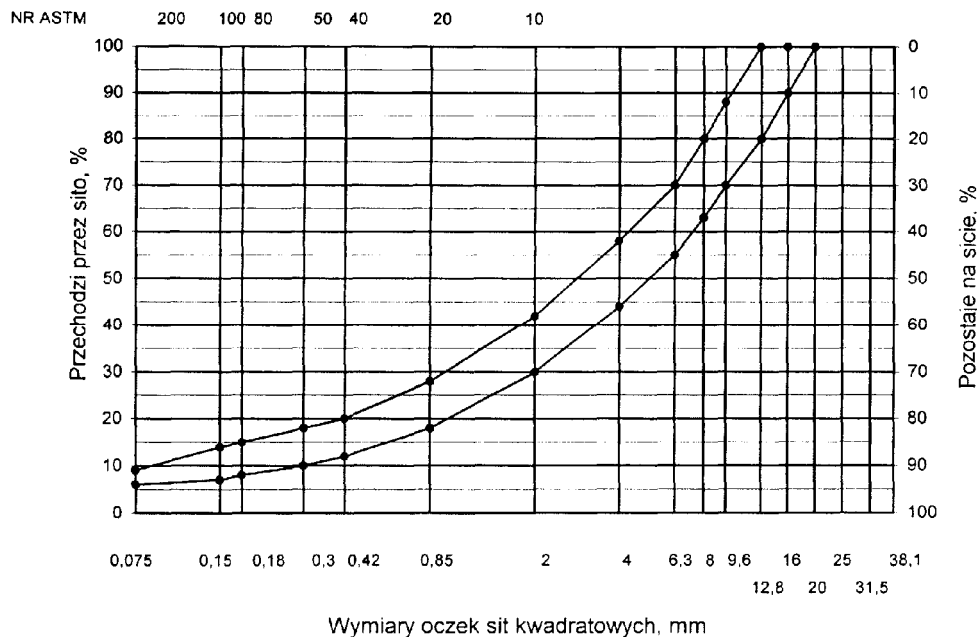
Rys. 2. Krzywe graniczne uziarnienia mieszanki mineralnej BA od 0 do 16 mm do warstwy ścieralnej nawierzchni drogi o obciążeniu ruchem KR3
