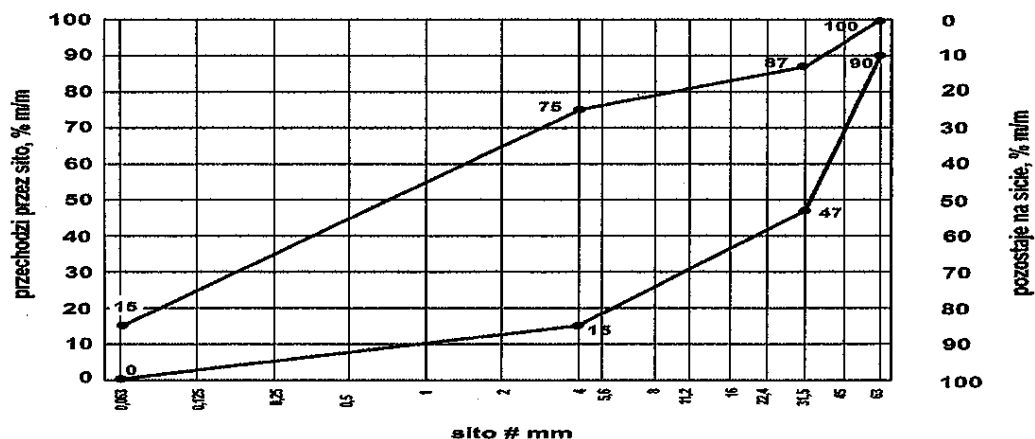
Rys. 7. Krzywe graniczne uziarnienia mieszanki kruszywo 0/63 mm do górnéj warstwy podłóža ulepszonego
