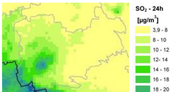
Rozkład stężeń SO 2 -24h w rejonie powiatu wołomińskiego (źródło: WIOŚ Warszawa 2015)
