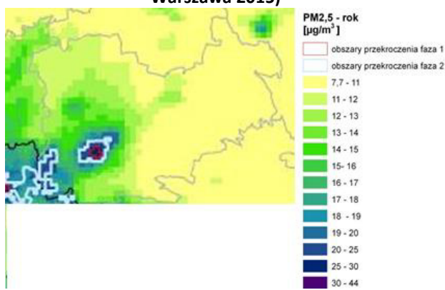
Rozkład stężeń PM2,5- rok (źródło: WIOŚ Warszawa 2015)
