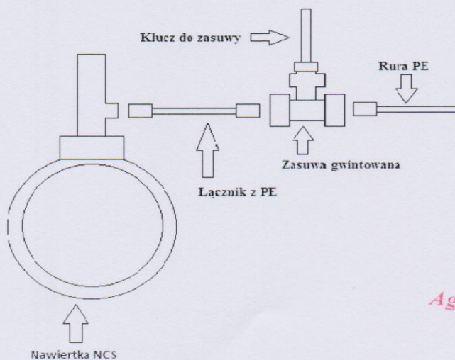
Schemat włączenia przyłącza do sieci wodociągowej
